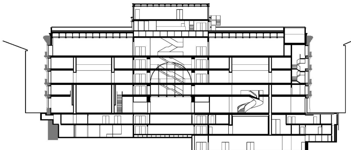
Corte seccional de Faro Santander. Cortesía de David Chipperfield Architects
